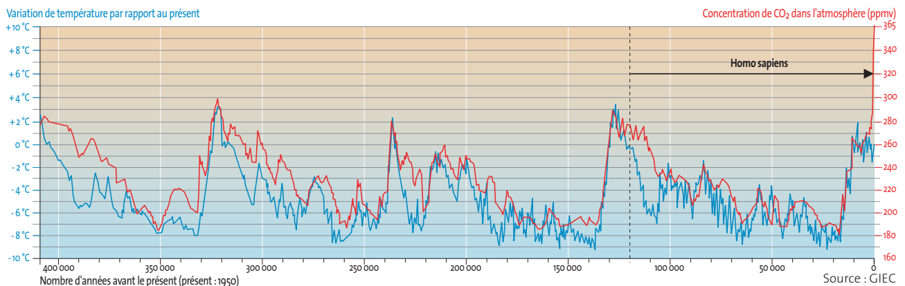
Graphique 1 : Evolution des températures de l’air et de la concentration en CO 2 durant les 400 derniers millénaires
