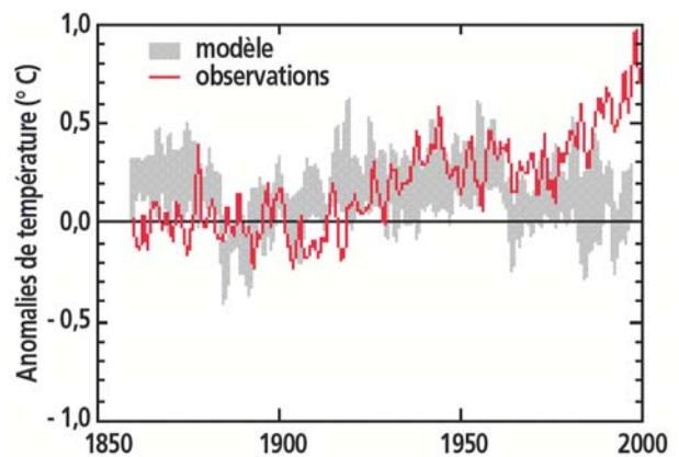
Graphique N° 5 : Températures à la surface simulées et moyennées annuellement et globalement.
