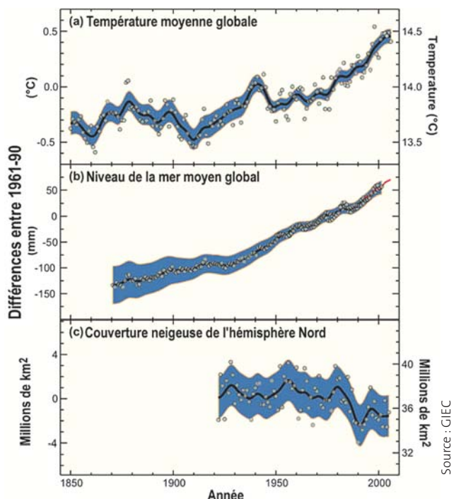
Graphique N° 3 : Variation de la température, du niveau de la mer et de la couverture neigeuse de 1850 à nos jours.
