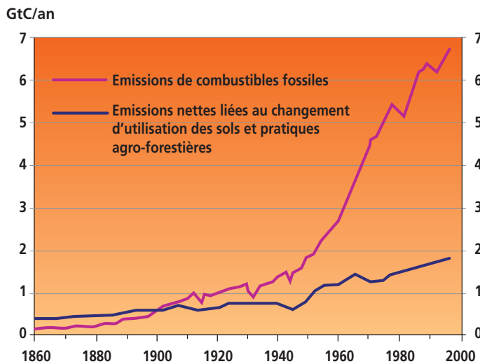
Graphique N° 6 : Les deux branches du carbone d'origine anthropique
