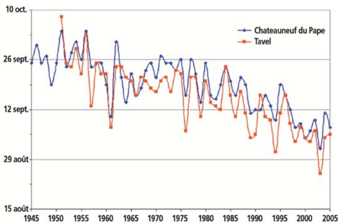
Graphique N° 4 : Dates de vendanges en Côtes du Rhône méridionales (appellations Châteauneuf du Pape & Tavel).
